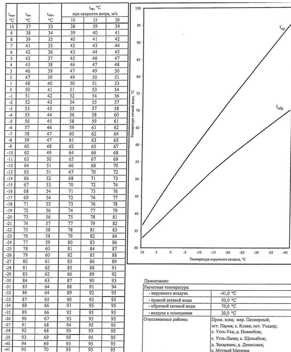
Рисунок 1.3.2 – Температурный график котельных с параметрами теплоносителя 95/70 °C на отопительный период 2020-2021 гг.
