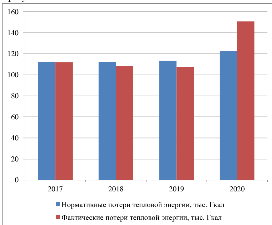
Рисунок 1.3.1 – Динамика тепловых потерь в период 2017-2020 гг. в тепловых сетях ООО «Усинская ТК»
