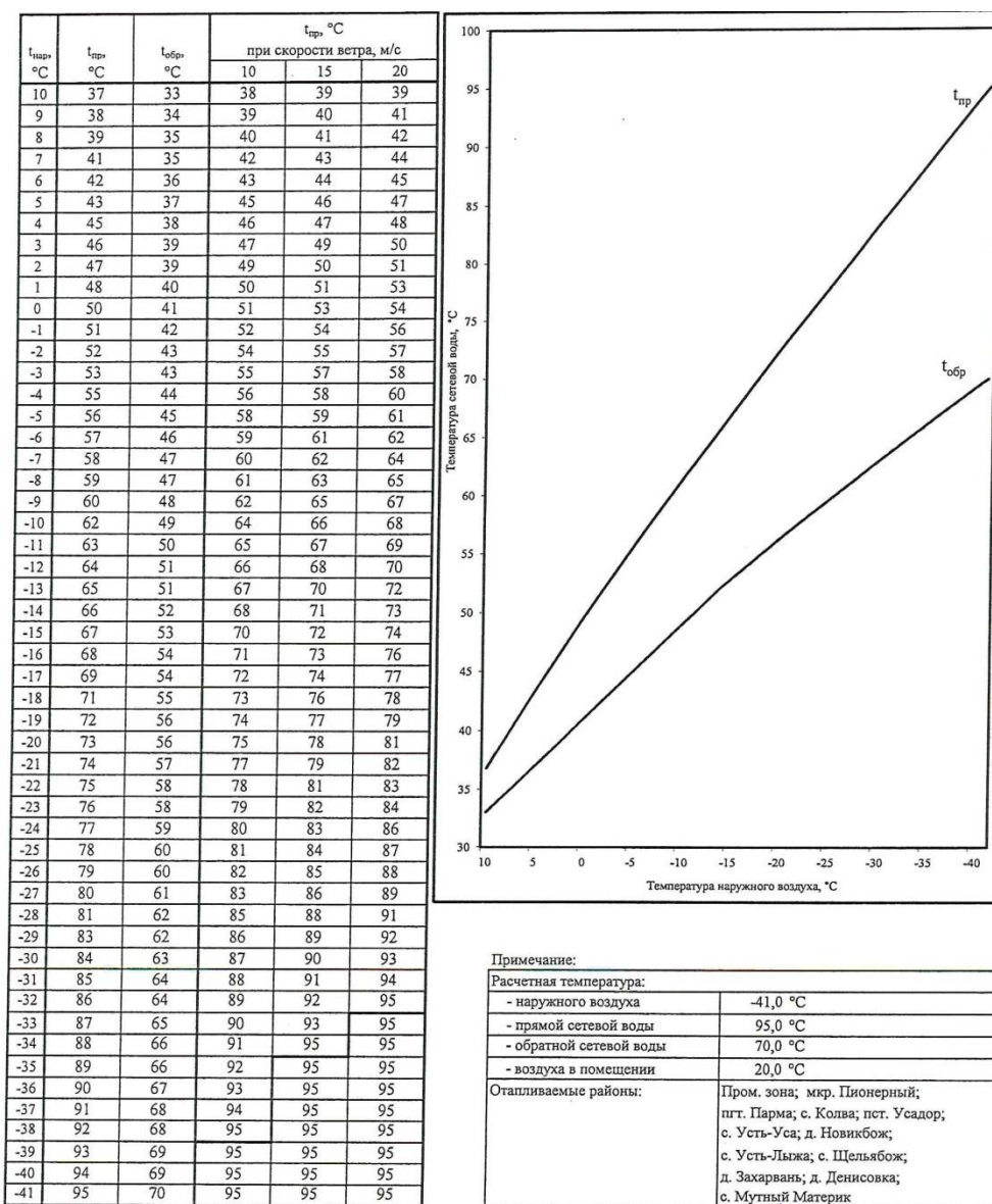
Рисунок 5.2 – Температурный график котельных и ТП «Пионерный» с параметрами теплоносителя 95/70 °C на отопительный период 2021-2022 гг.
