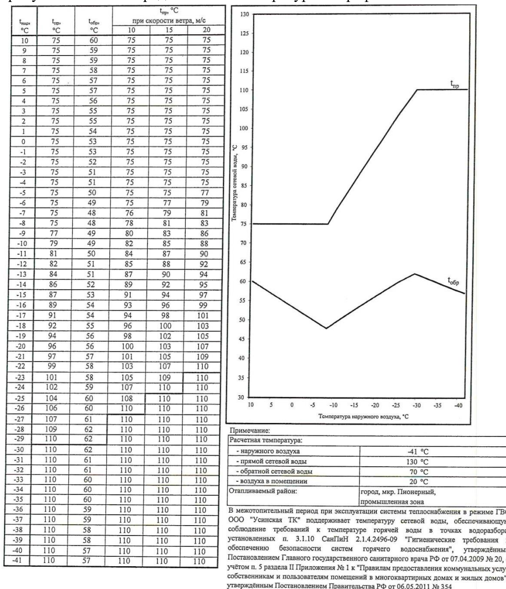
Рисунок 5.1 – Температурный график центральной водогрейной котельной с параметрами теплоносителя 130/70 °C со срезкой на 75 и 110 °C на отопительный период 2021-2022 гг.
